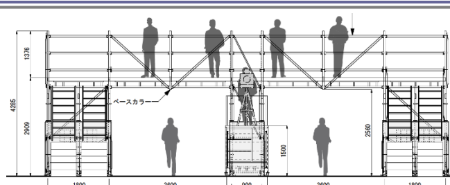
フォトブリッジ(正面図)
