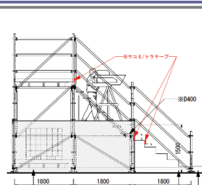
フォトブリッジ(側面図)
